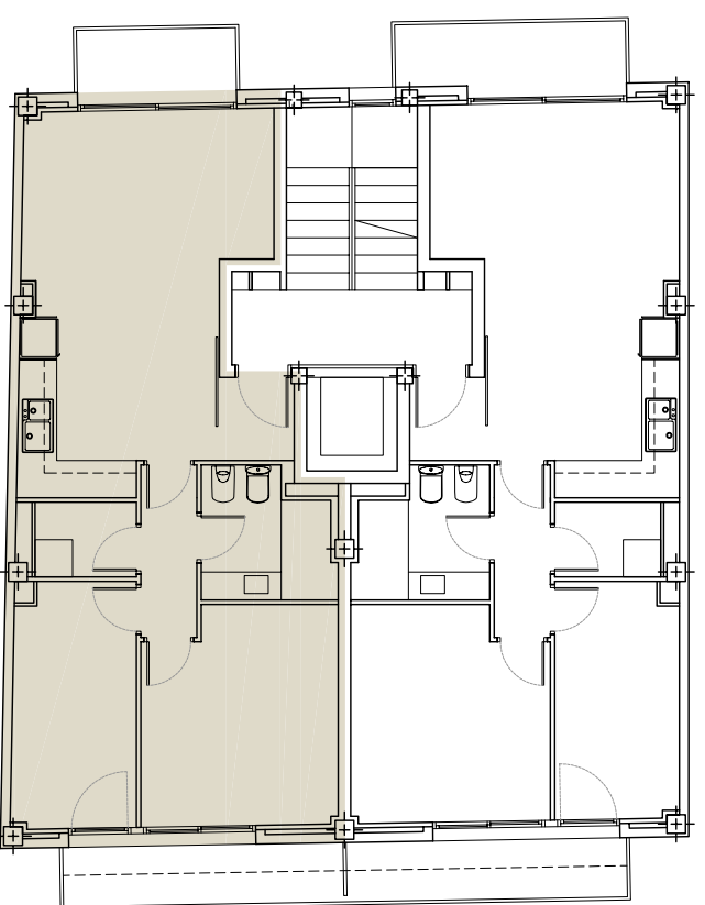
PLANTA PRIMERA I SEGONA
